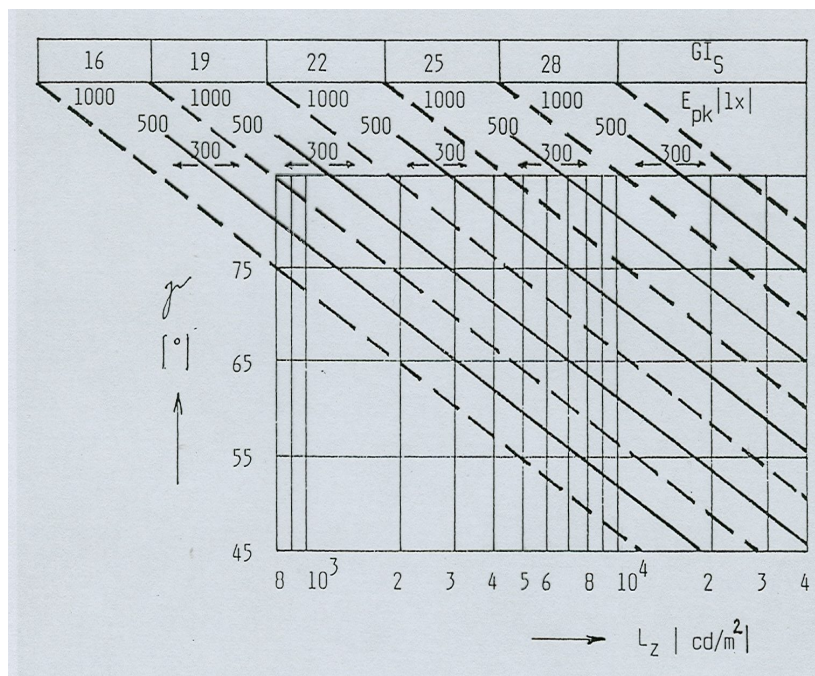
Obr.8-7 Diagram s čarami mezních jasů v systému UGR pro pravoúhlé prostory s rovnoměrně rozmístěnými svítidly, jejichž vyzařování popisují typové charakteristiky BZ
