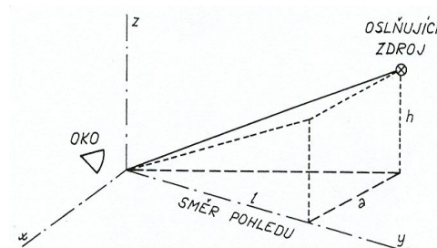
Obr.8-6a Geometrické uspořádání pro stanovení činitele polohy P z diagramu na obr.8-6
