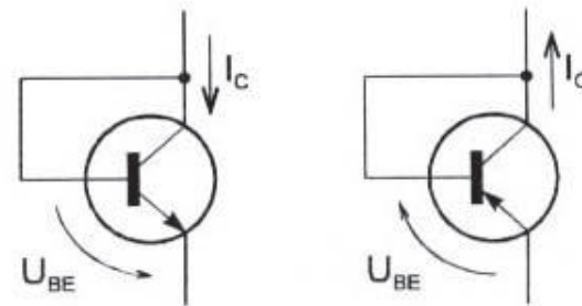
Tranzistorová dioda
