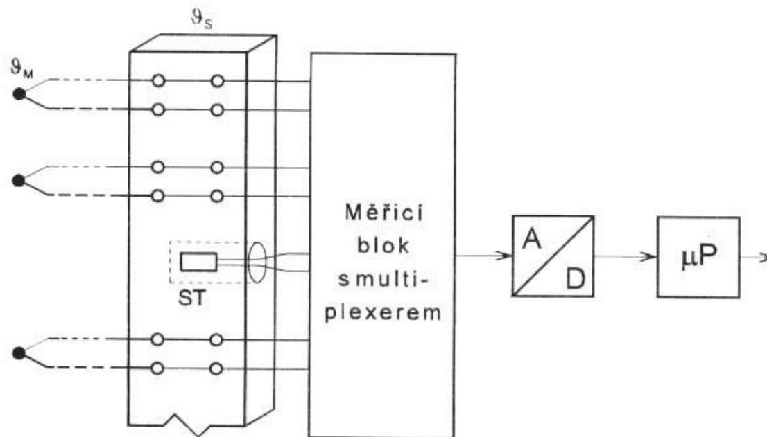
Obr. 3.33 Izotermická svorkovnice
