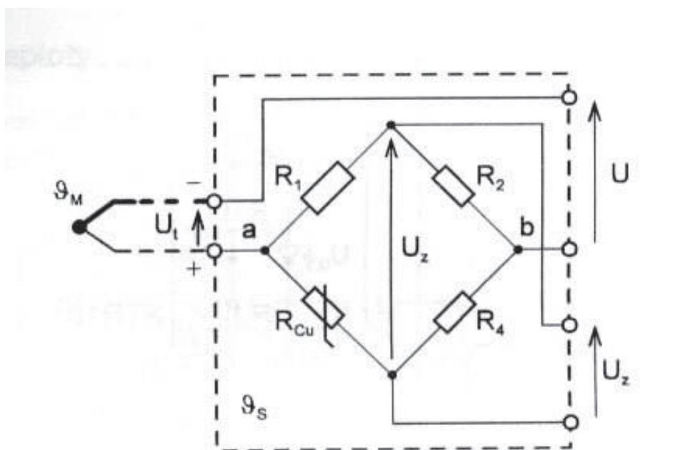
Obr. 3.30 Zapojení kompenzační krabice
