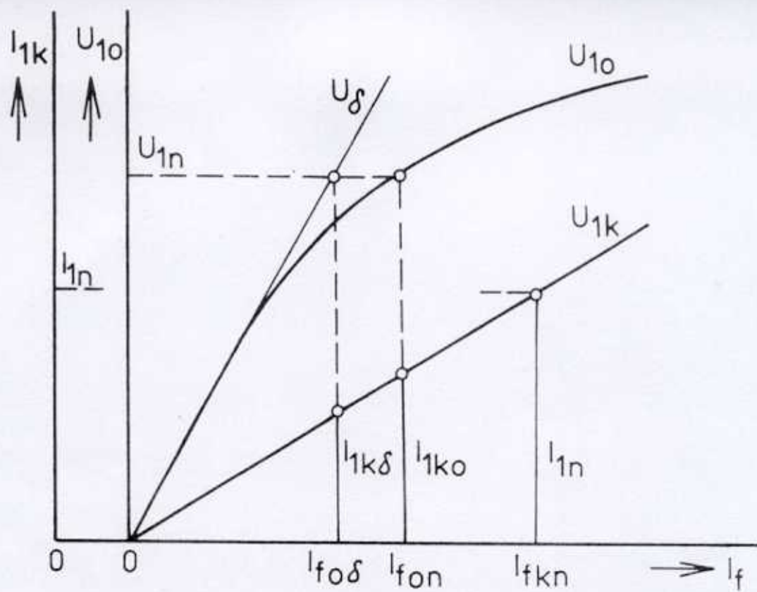
Obr. 10-1 Charakteristika naprázdno a nakrátko
