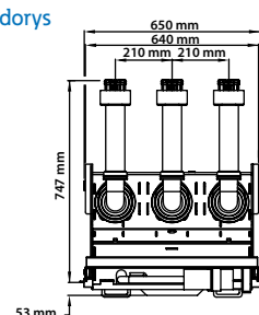
Půdorys
