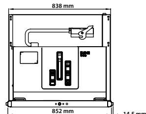
Nárys
