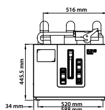
Nárys
