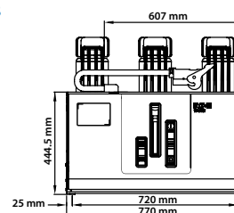
Nárys
