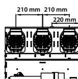
Půdorys
