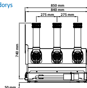
Půdorys
