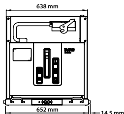
Nárys
