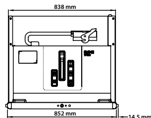
Nárys
