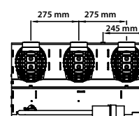
Půdorys
