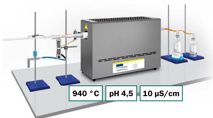
Korozivita vzniklých plynů dle ČSN EN 60754-2
